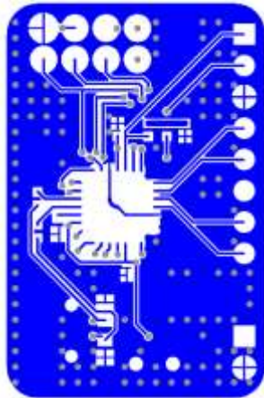
Bottom Layer
